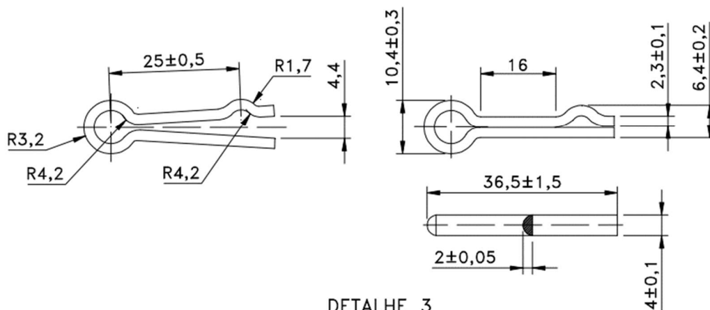
DETALHE 3 DIMENSÕES CUPILHA
