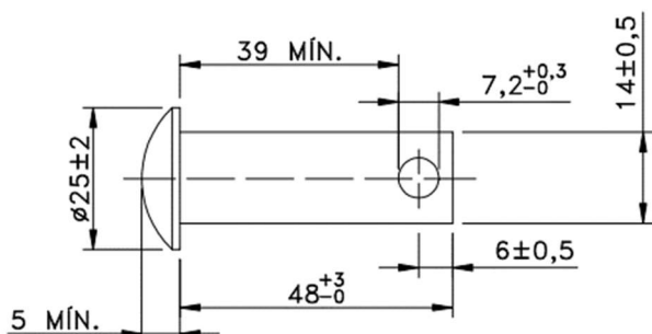
DETALHE 1 DIMENSÕES PINO 1
