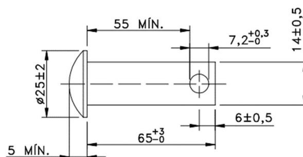
DETALHE 2 DIMENSÕES PINO 2
