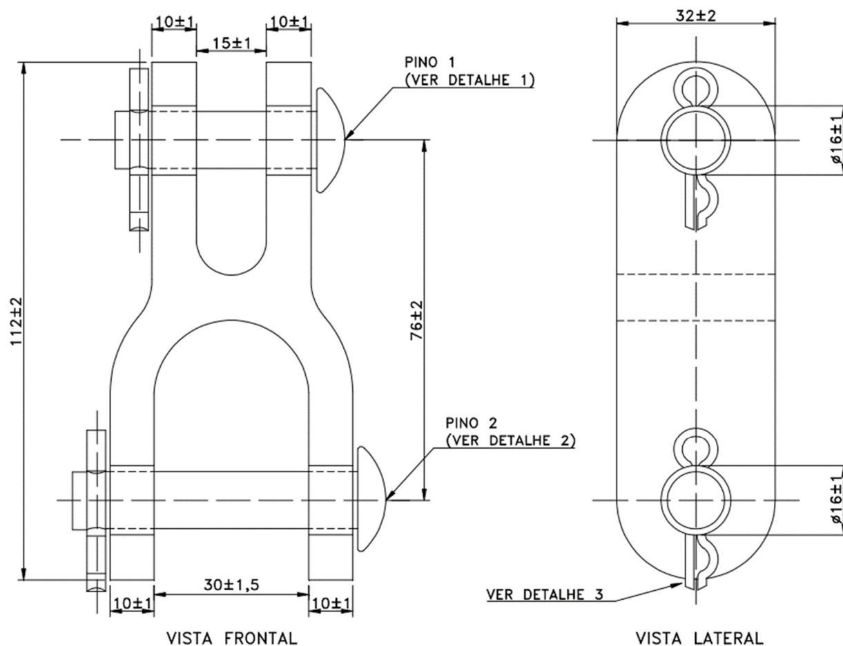
Figura 1 – Vista frontal e lateral do Garfo Duplo
